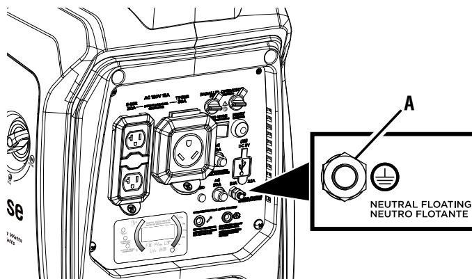
A - Terminal de tierra
