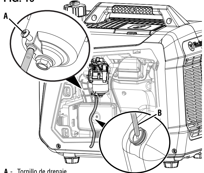
A - Tornillo de drenaje B - Manguera de drenaje
