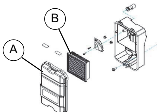
Figura 4-3. Conjunto del filtro de aire
