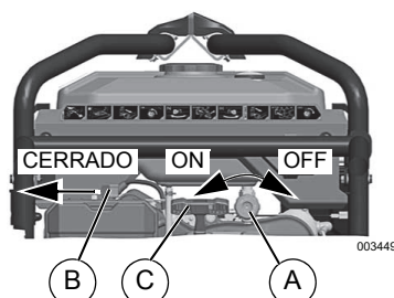
Figura 3-2. Controles del motor
