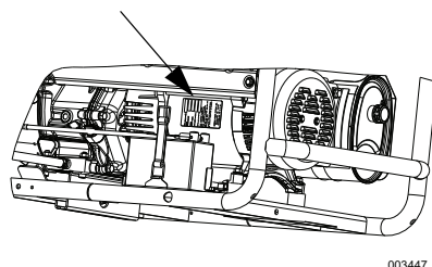
Figure2-2. Étiquette d'identification du produit
