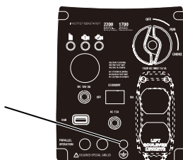
Figure 3-1. Mise à la terre du générateur
