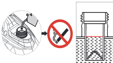
Figure 2-9. Niveau à l'intérieur du réservoir de carburant
