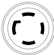
Figure 2-6. Prise de courant de 120/240 V c.a., 30 A
