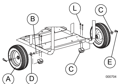
Figura 2-8. Conjunto de ruedas
