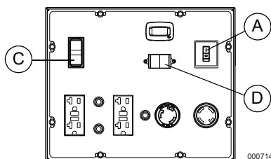
Figura 3-4. Conmutador Run/Stop (funcionamiento/parada) del motor
