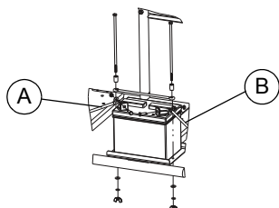
Figure 4-5. Raccordement de la batterie
