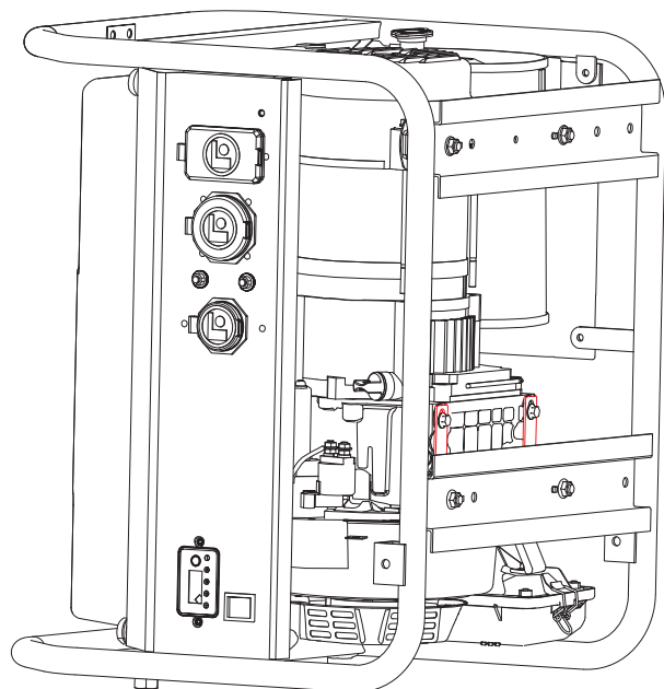
Soportes del Motores (Color rojo)
