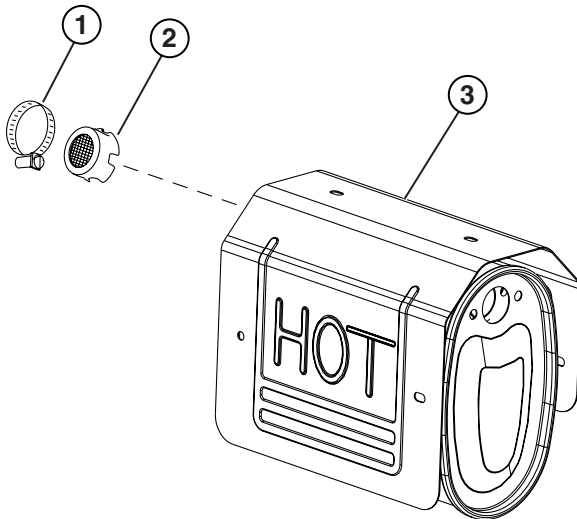
Figura 42 – Conjunto del amortiguador de chispas
