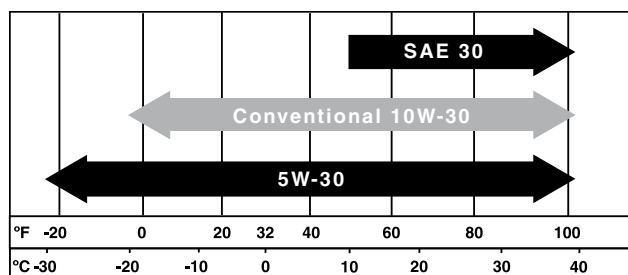
Figura 25 – Aceite recomendado
