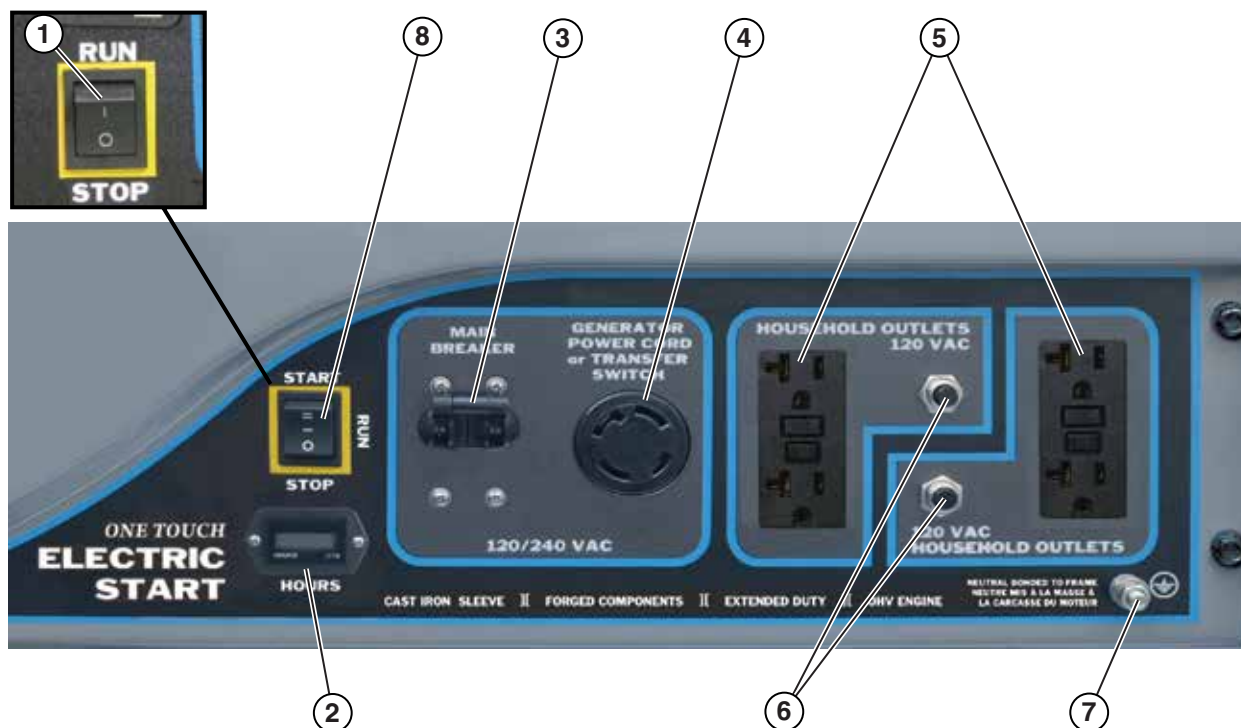
Figura 11 – Características del panel de control
