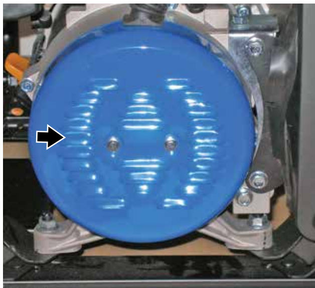
Figura 45 – Entrada de aire de refrigeración y orificio de escape del alternador
