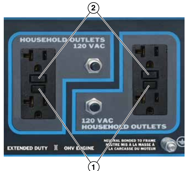
Figura 39 – Tomacorriente GFCI
